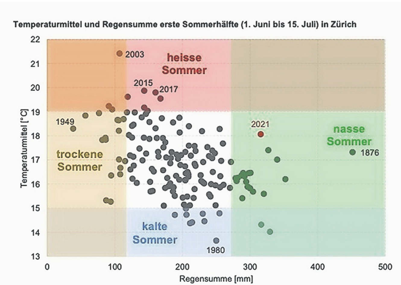
Einteilung der ersten Sommerhälften in Zürich von 1864 bis 2021 (jedes Jahr ein Punkt) bezüglich Regensumme und Temperaturmittel. Oben links sind heiss-trockene Sommer wie 2003. Die erste Sommerhälfte 2021 war äusserst nass (rechts im Diagramm), aber auch relativ warm (oben). GRAFIK ROS
